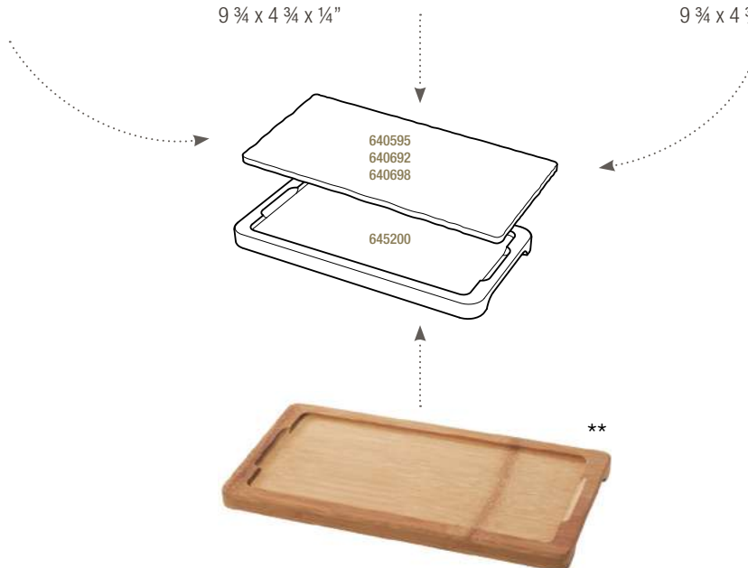
PLATEAU POUR PLANCHE 25 X 12 CM LINER TRAY FOR TRAY 9 3/4 x 4 3/4"
